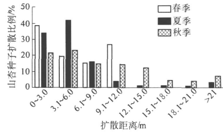
图 3 不同季节释放山杏种子扩散距离的频度分布
